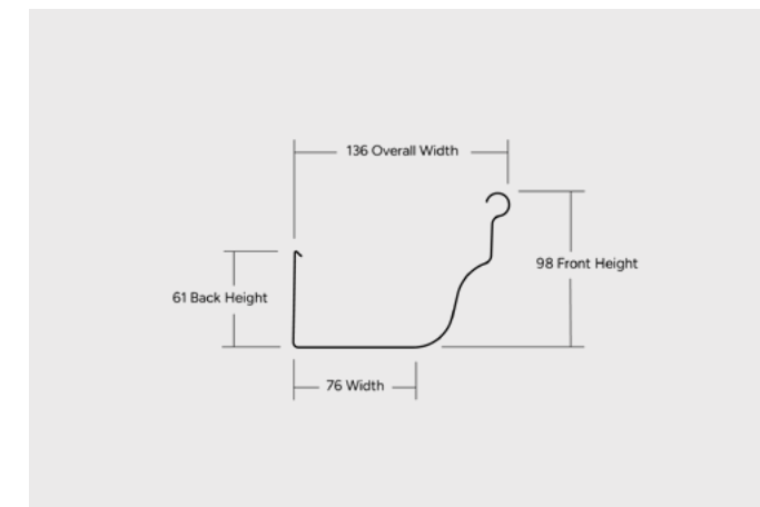
O-GEE GUTTER (SA)
