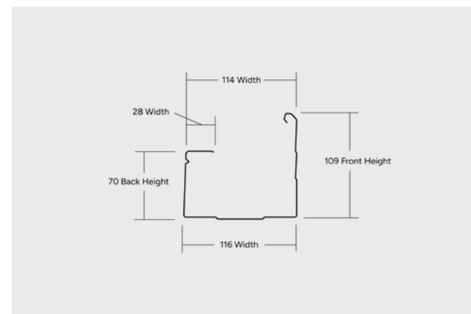
EASLINE DOMESTIC (WA)
