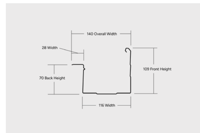
EASLINE PATIO (WA)
