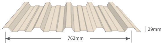
Stramit Monoclad®
