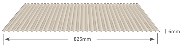
Stramit Mini Corry®
