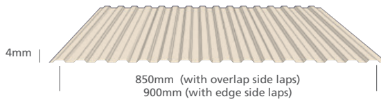
Stramit Minirib®
