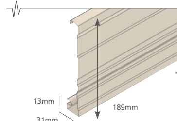
Stramit® Metal Fascia
